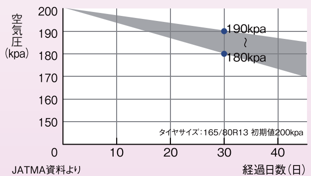
経過日数と空気圧の減り方
